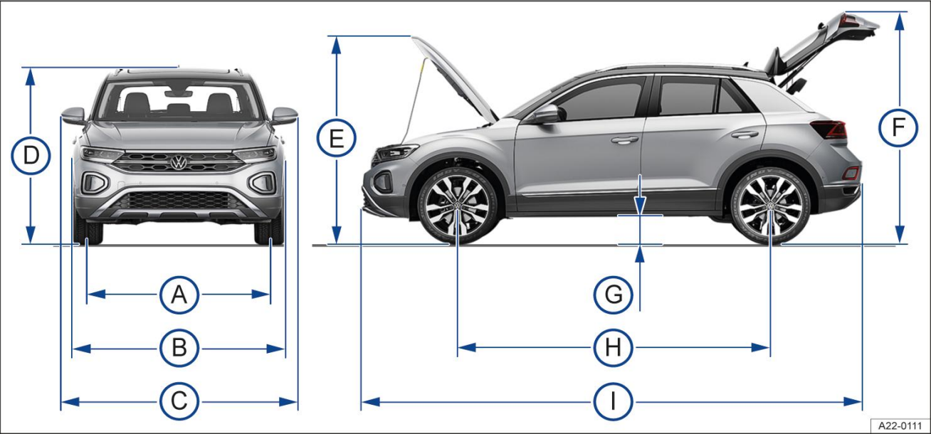
Фиг. 1 Размери на автомобила
